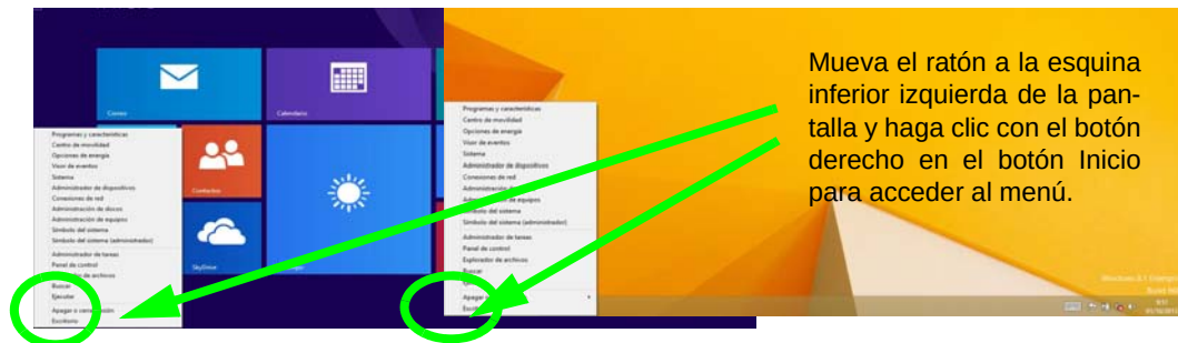
Figura 6 Menú contextual
