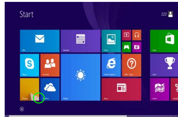
Abb. 7 - Start-Bildschirm
