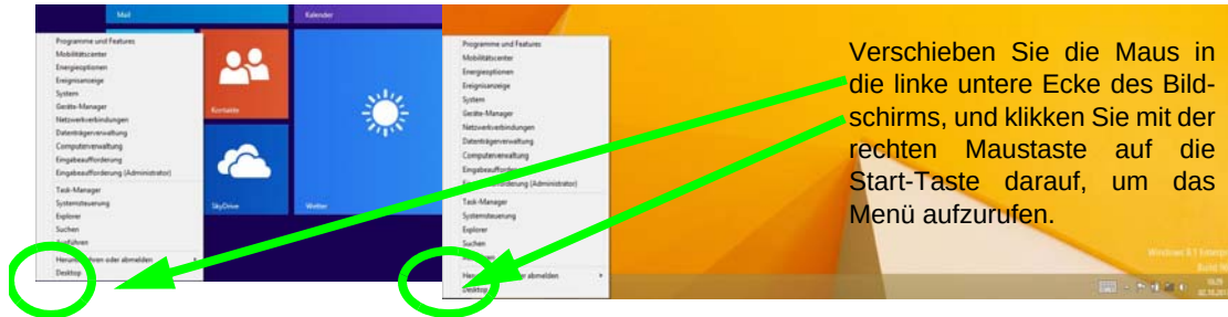
Abb. 6 Kontextmenü
