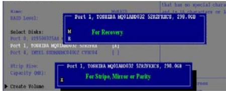
Abb. 3 Ausgewählte Festplatten
