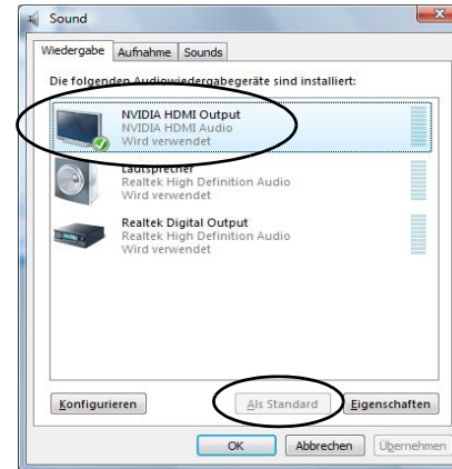
Abb. 17 Klangwiedergabeoptionen
