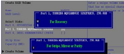
Figure 3 Sélectionnez disques
