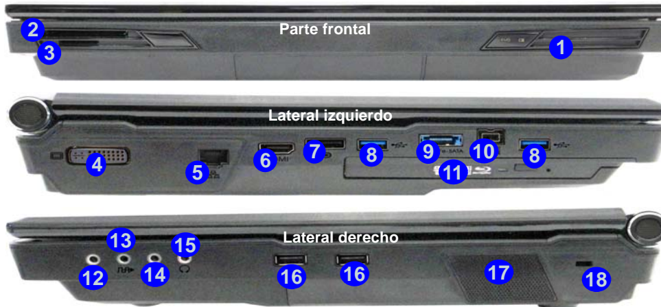
Figura 9 Vistas frontal, izquierda y derecha
