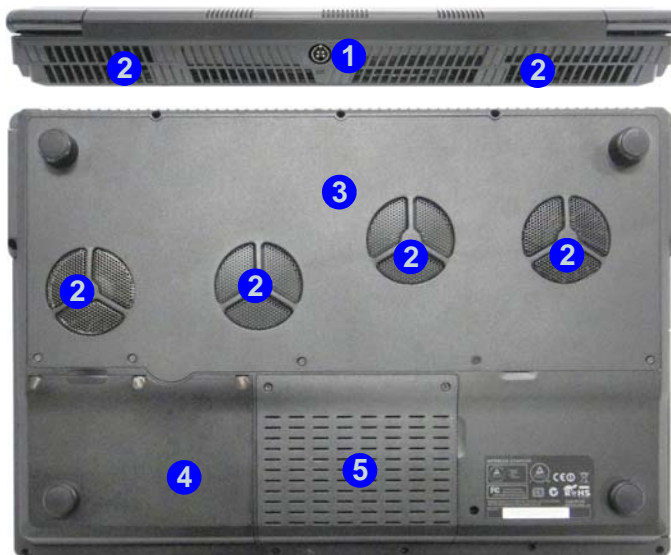
Figura 10 Vista posteriore e inferiore
