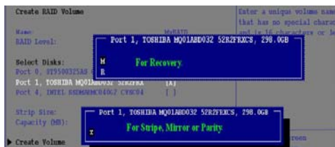
Figura 3 Scegliere dischi
