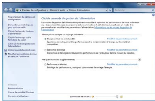
Figure 15 - Options d'alimentation
